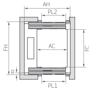
2 TOEGANGEN (TEGENOVERLIGGEND)
