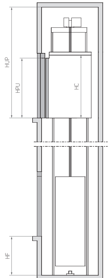
VERTICALE DOORSNEDE
